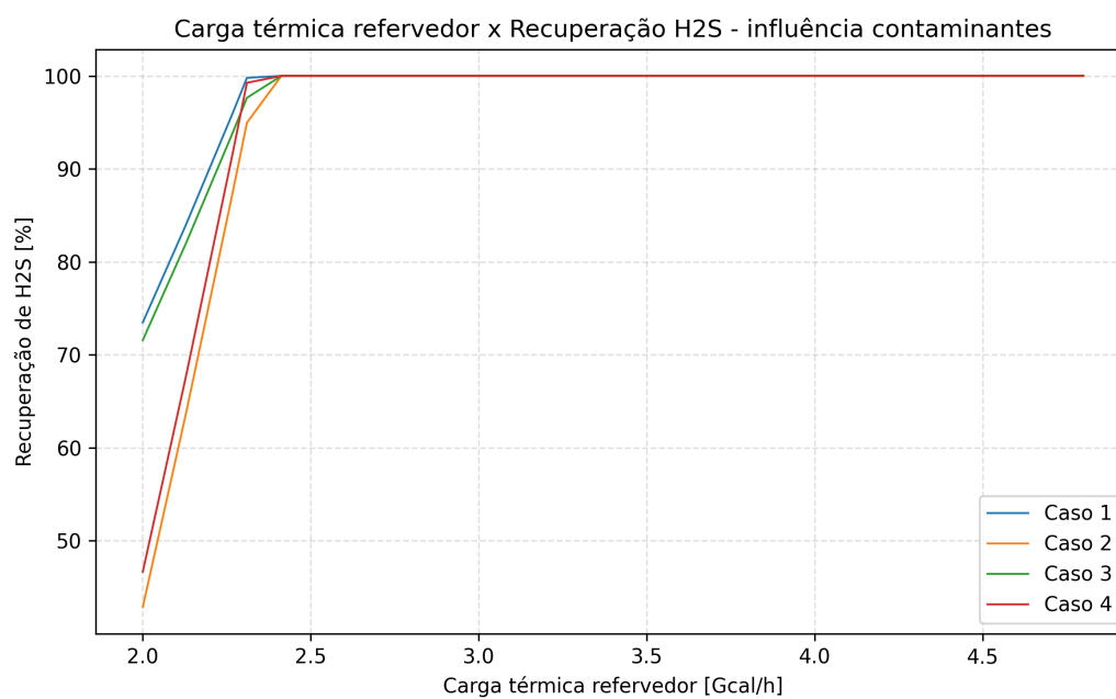
Figura 5: Carga térmica x recuperação de H 2 S - Influência Contaminantes
