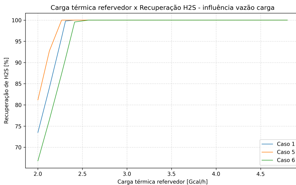
Figura 13: Carga térmica x recuperação de H 2 S - Influência Vazão da Carga
