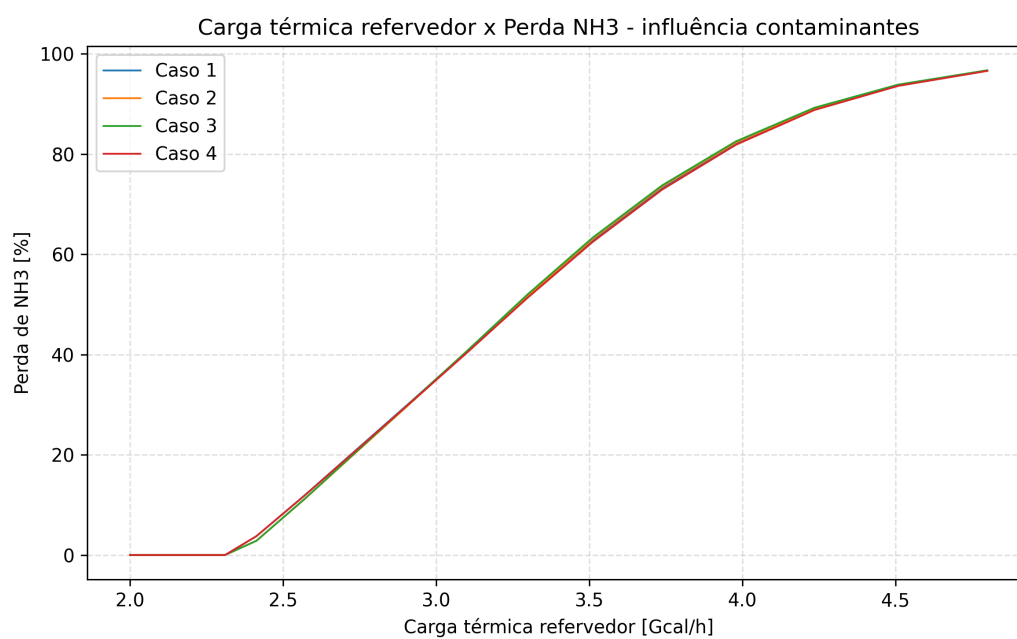
Figura 6: Carga térmica x perda de NH 3 - Influência Contaminantes
