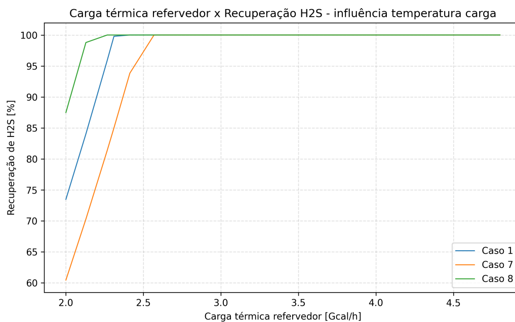
Figura 9: Carga térmica x recuperação de H 2 S - Influência Temperatura da Carga
