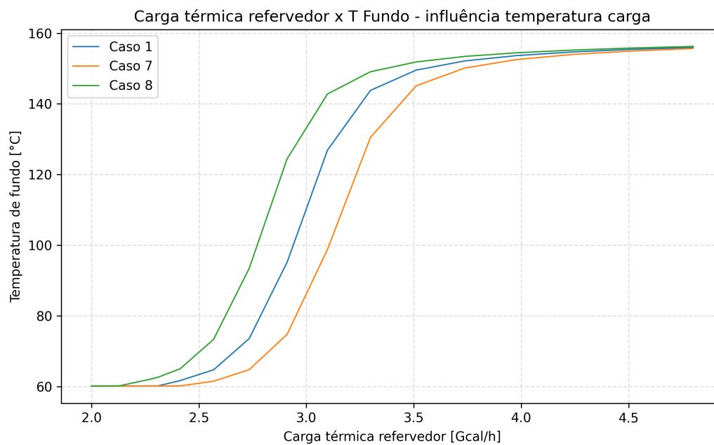
Figura 11: Carga térmica x temperatura do fundo - Influência Temperatura da Carga
