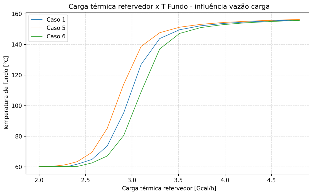
Figura 15: Carga térmica x temperatura do fundo - Influência Vazão da Carga
