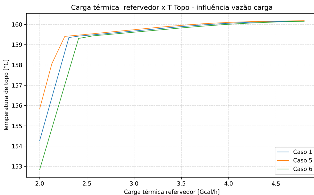
Figura 16: Carga térmica x temperatura do topo - Influência Vazão da Carga
