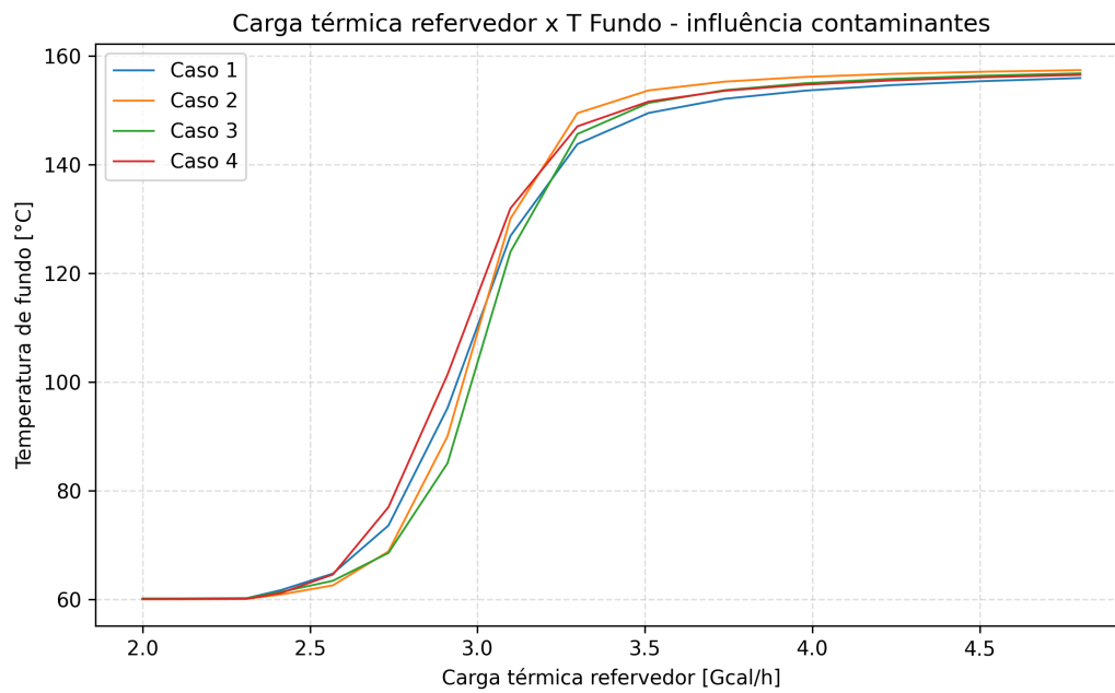
Figura 7: Carga térmica x temperatura do fundo - Influência Contaminantes
