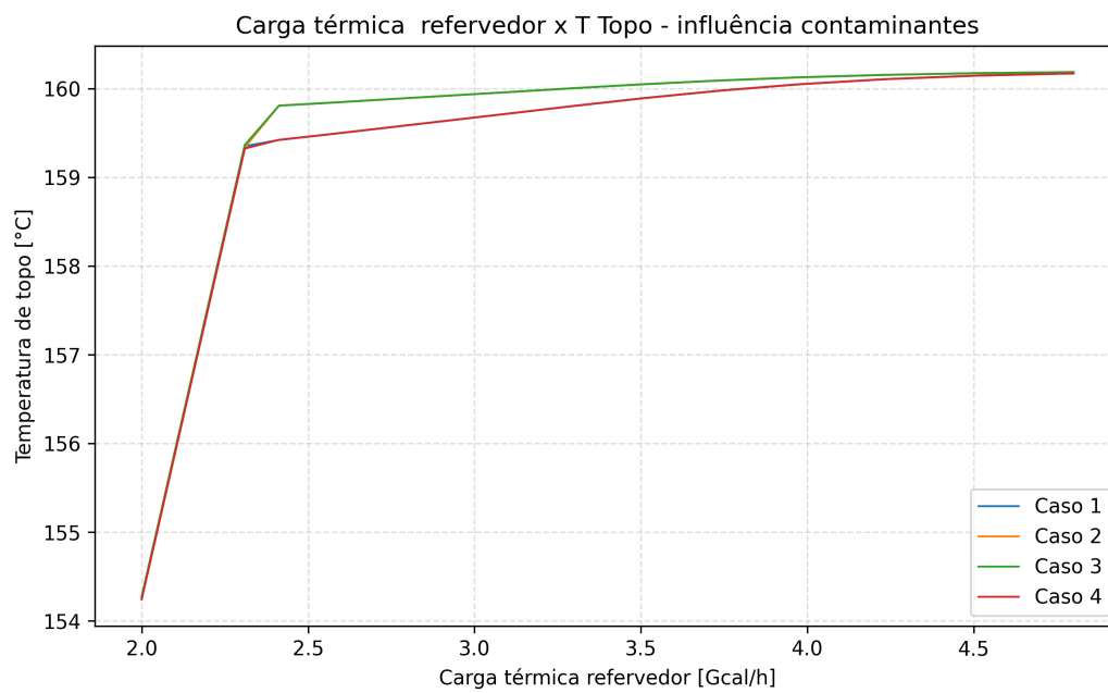
Figura 8: Carga térmica x temperatura do topo - Influência Contaminantes
